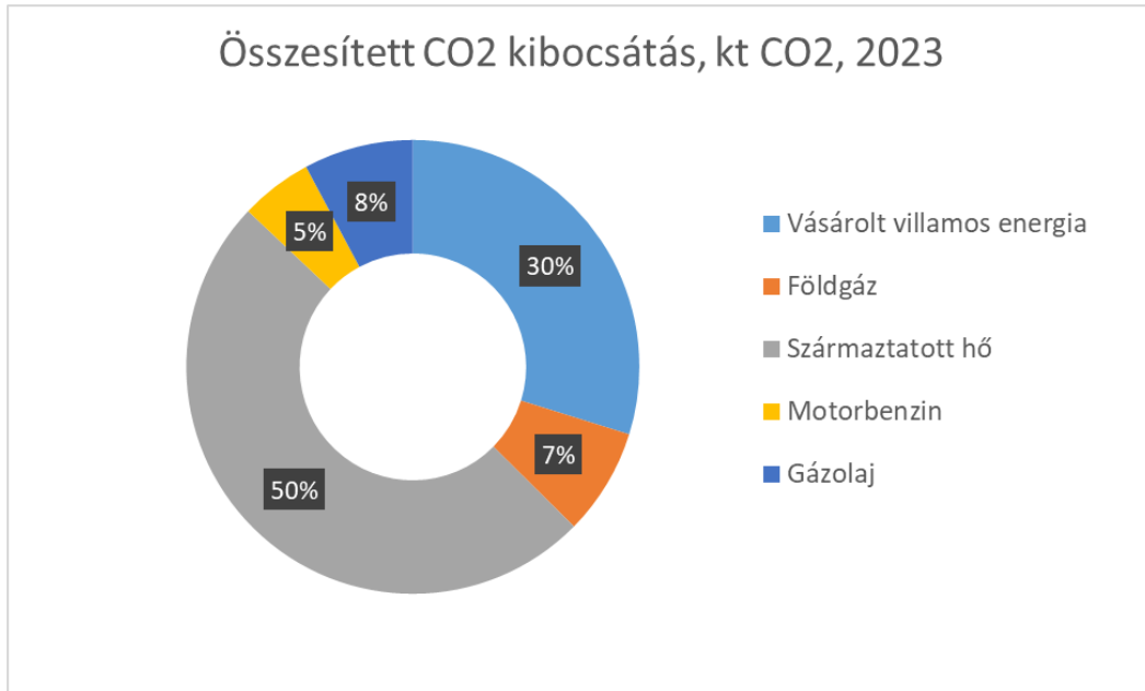
2. Ábra A Társaság összesített CO 2 kibocsátása energiahordozónként
